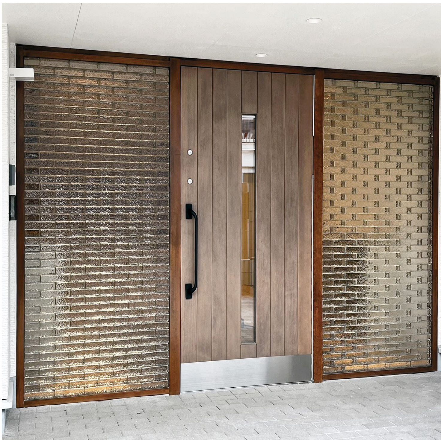
※旧型 WAVE 施工例
